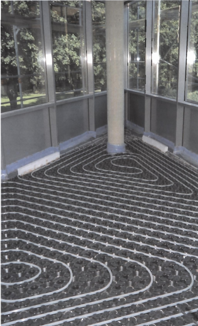
verlegter proKLIMA Systemboden mit Rohbaumontageblock und Systemrohr
